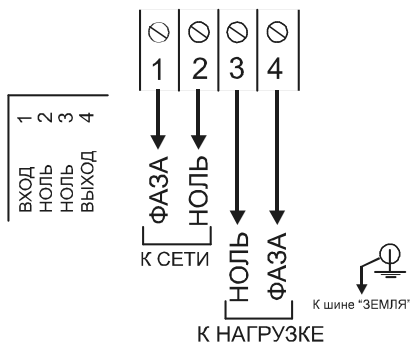
Рис.3. Подключение стабилизатора к сети и к нагрузке
