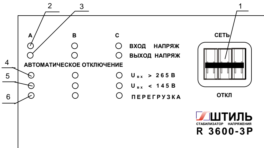
Рисунок 4.1 Передняя панель стабилизатора
